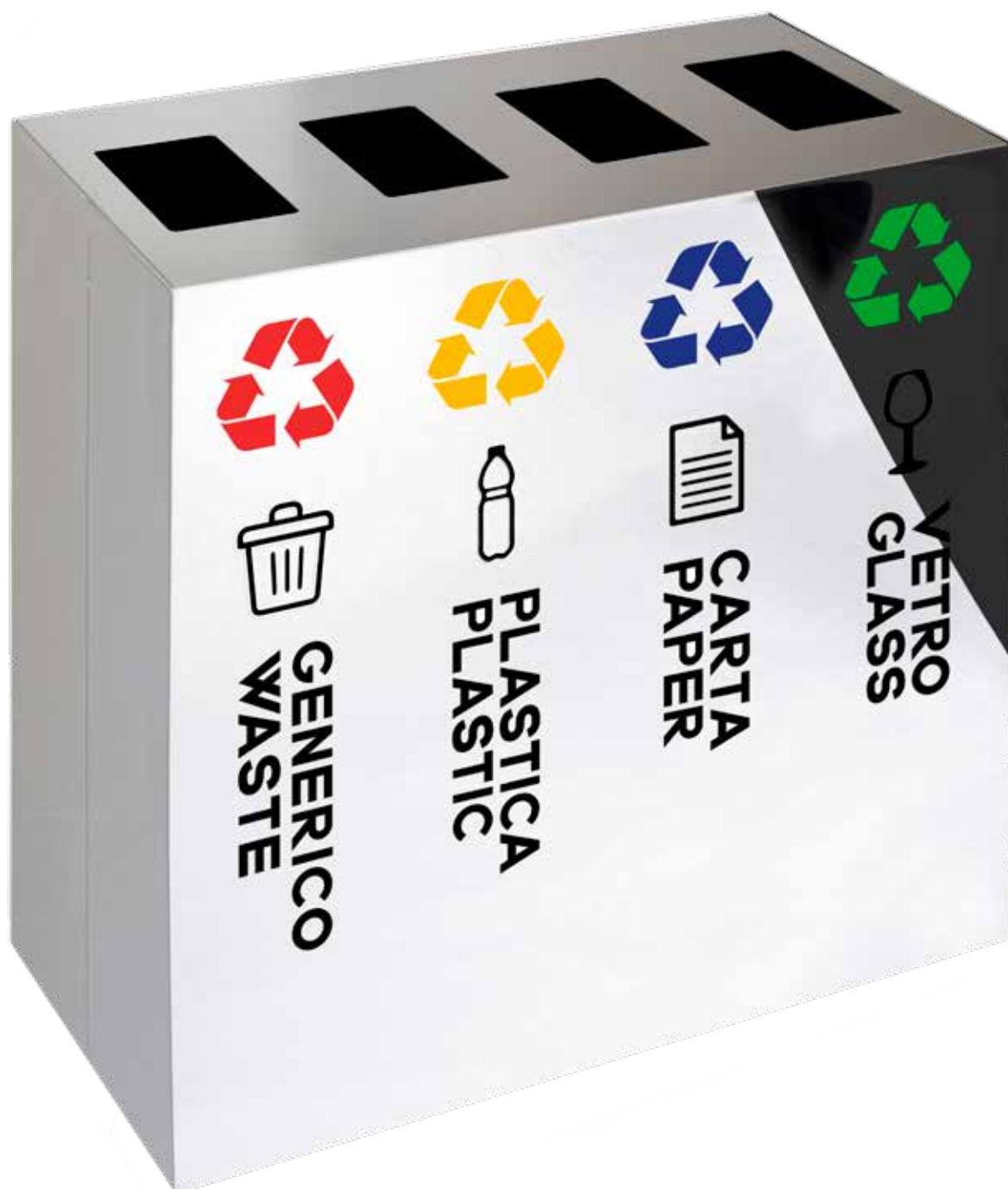
584/A - SOLUZIONE A CONTENITORE IN ACCIAIO INOX PER RACCOLTA DIFFERENZIATA CON COPERCHIO E ANELLO REGGISACCO A QUATTRO SCOMPARTI STAINLESS STEEL CONTAINER FOR SEPARATE WASTE COLLECTION WITH LID AND BAG RING FOUR COMPARTMENTS 30 x 60 x H 67 cm - LITRI 4 x 30
